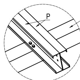
DETAL C5
