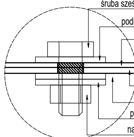
DETAL C6
