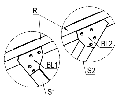
DETAL C5
