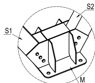
DETAL C1
