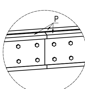
DETAL C3
